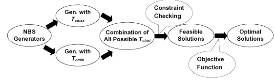
Fig. 5. Enumerative algorithm.
